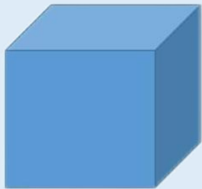
正方体
